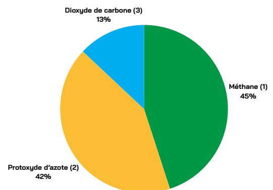
Figure 1 : Emissions de GES du secteur agricole (1)
